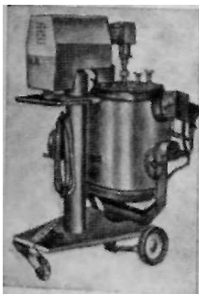
Рис. 4. Машина для приготовления картофельного пюре МКП-60
