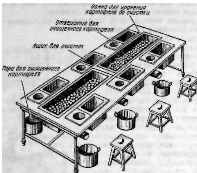
Рис. 14. Стол для доочистки картофеля
