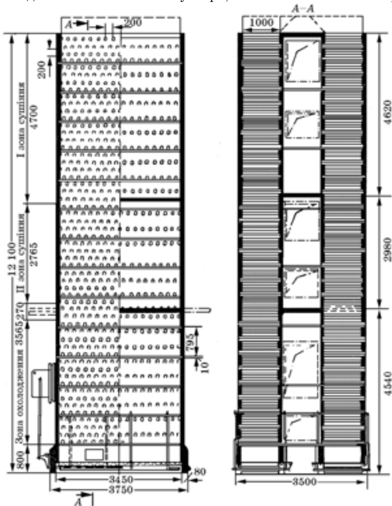
Рис. 8. Шахтна зерносушарка
