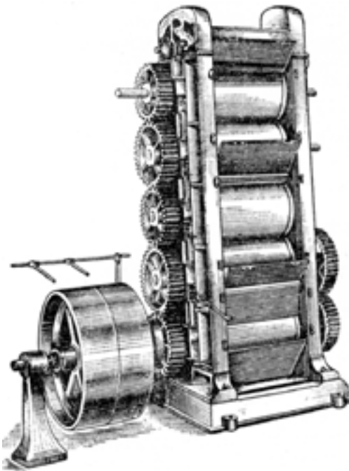
Рис. 16. П'ятивальцовий верстат
